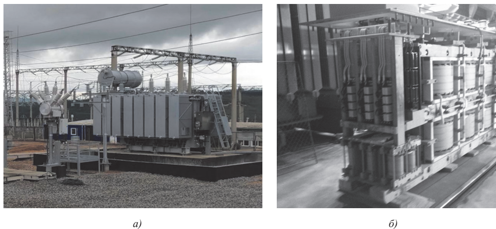
Рис. 6. УШРТм мощностью 25 МВ·А напряжением 35 кВ (полная масса 52 т, номинальные потери 200 кВт; габариты: длина 6460 мм, ширина 3565 мм, высота 4900 мм): a – общий вид; б – выемная часть
